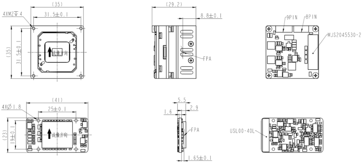
图 1. LV0625A 机械接口与外形尺寸
