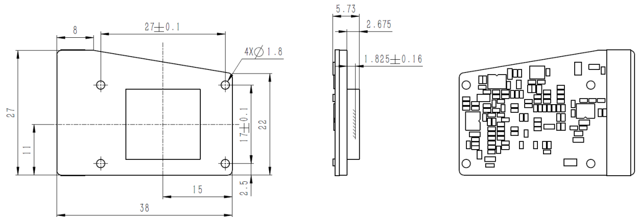
图6. 可见光组件机械外形与接口尺寸
