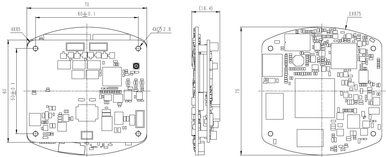
图7. 处理板 + 接口板机械外形与接口尺寸
