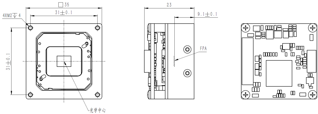
图5. 红外组件机械外形与接口尺寸
